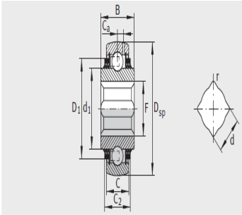
GVK..-KTT-B(-AH..)-AS2/V, VK..-KTT-B(-AH..)
