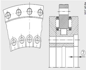
对于 YRT80-TV 和 YRT100 : ② 螺栓沉头孔开口方向 5)
