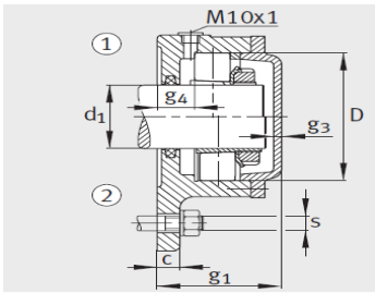
设计类型 A ① 定位轴承 ② 浮动轴承
