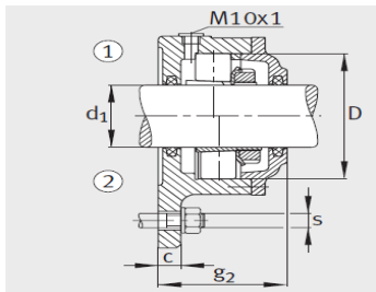
设计类型 B ① 定位轴承 ② 浮动轴承
