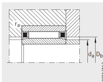
滚针和保持架组件 在轴承座里的轴向引导
