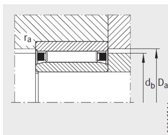
滚针和保持架组件 在轴上的轴向引导
